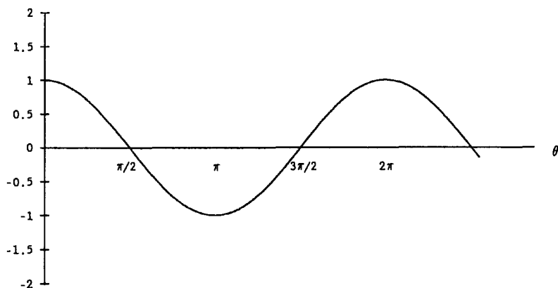
(b) \cos(\theta)
