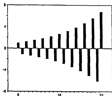
(d) \phi = -1.1
